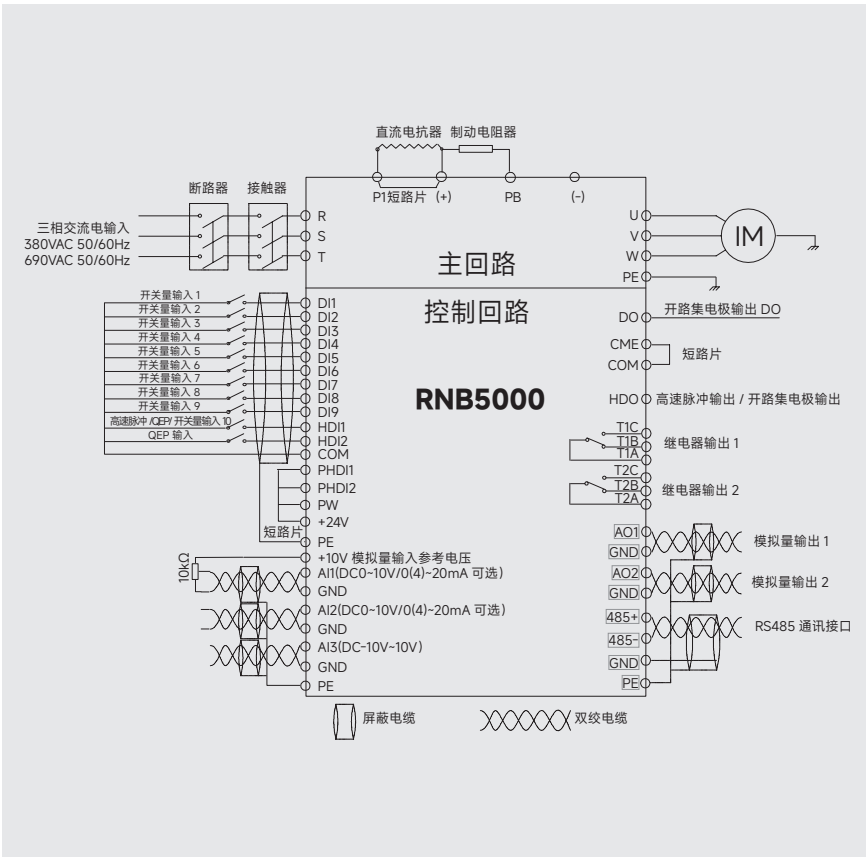
图 3-7 标准接线图
