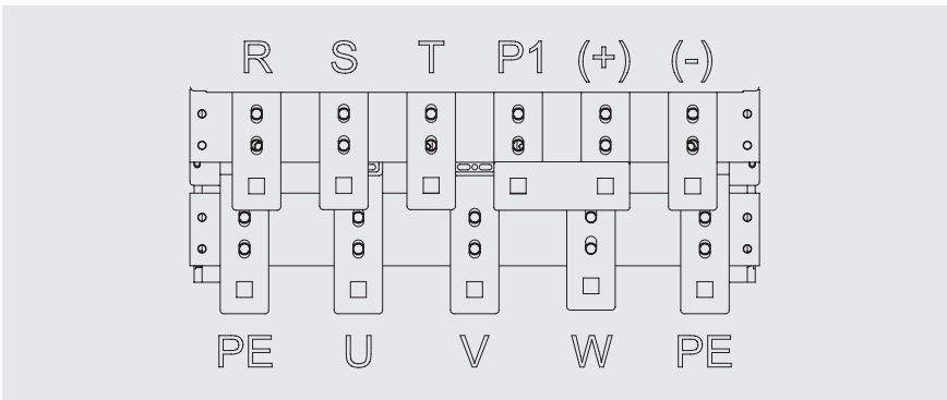
图 3-4 RNB5160-6T ~ RNB5220-6T 主回路接线端子图
