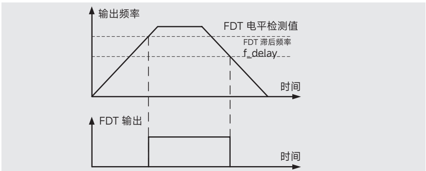
图 6-20 输出频率与 FDT 输出关系图
