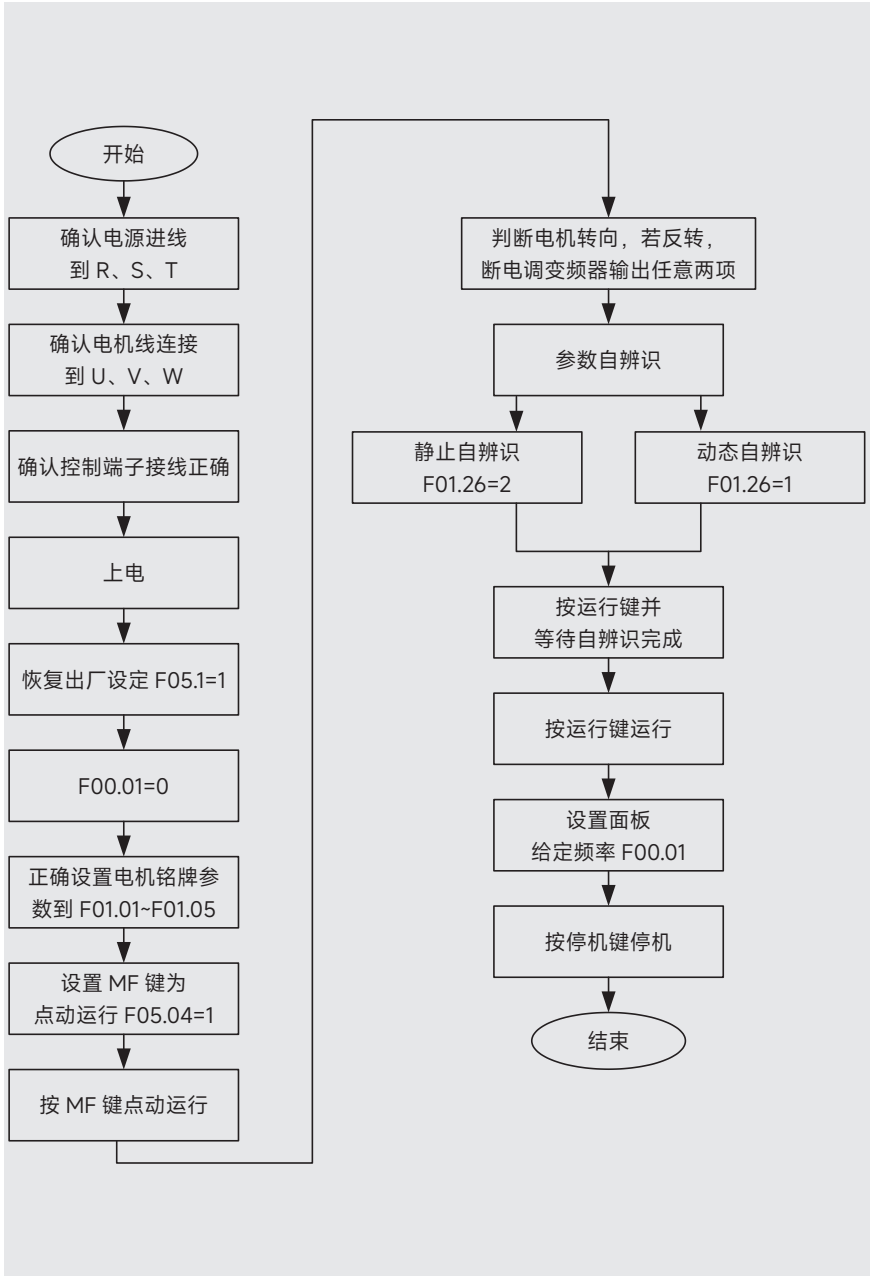
图 4-2 首次上电流程图
