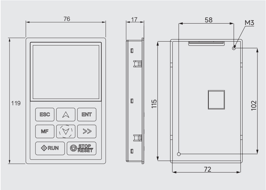
图 2-4 面板外形及尺寸图 (单位 mm)
