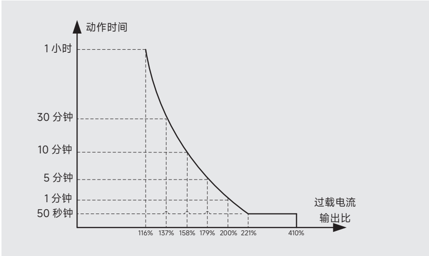
图 6-1 过载保护动作时间与电流比的关系
