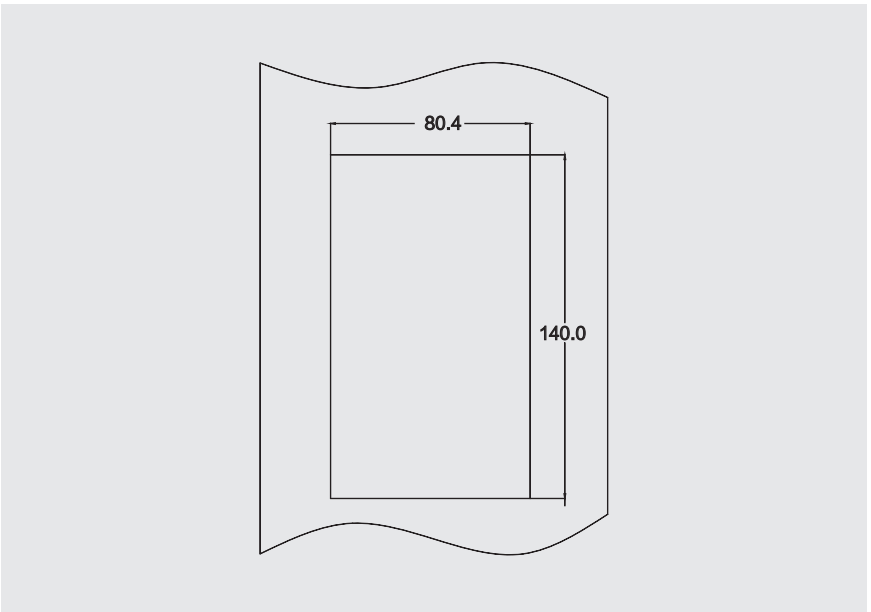
图 2-7 操作面板支架外引开孔尺寸图
