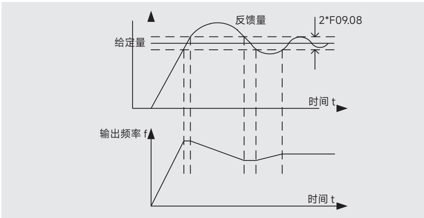
图 6-16 过程 PID 控制示例
