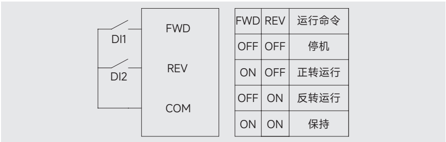
图 6-9 两线式控制 1
