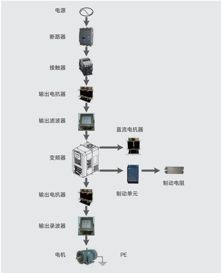
图 3-1 产品外围元器件的标准配置图
