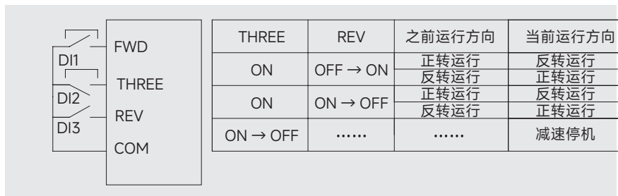
图 6-11 三线式控制 1
