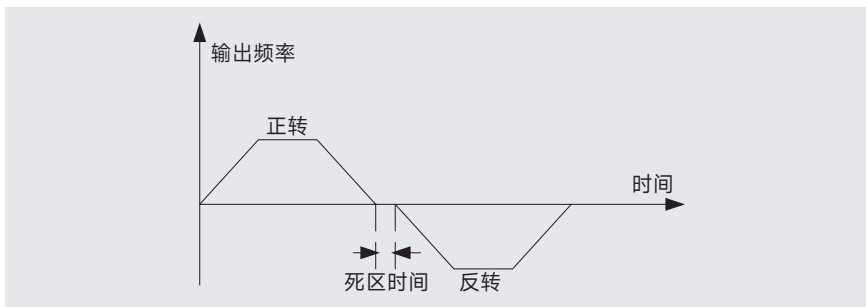
图 6-3 正反转死区时间示意图
