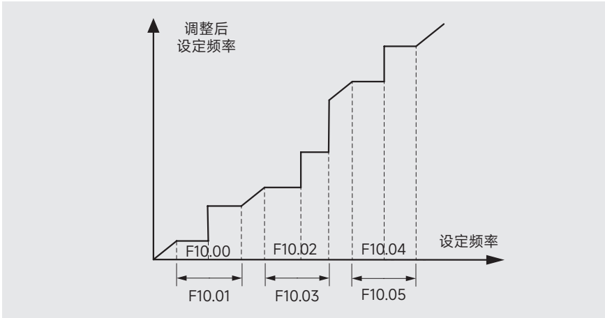
图 6-17 跳跃频率处理
