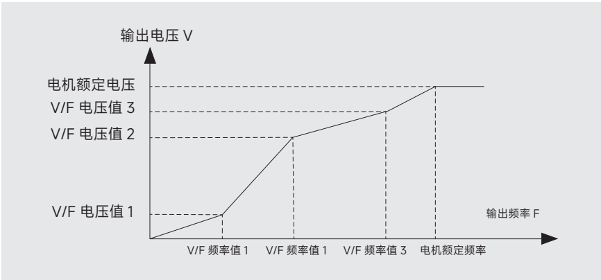
图 6-6 多点 V/F 曲线图
