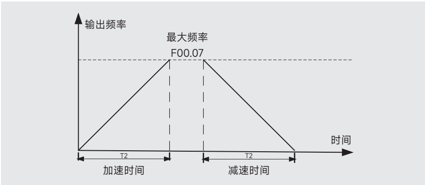
图 6-2 恒加减速曲线图
