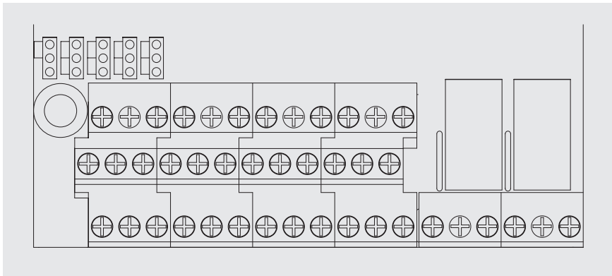
图 3-9 控制板端子示意图
