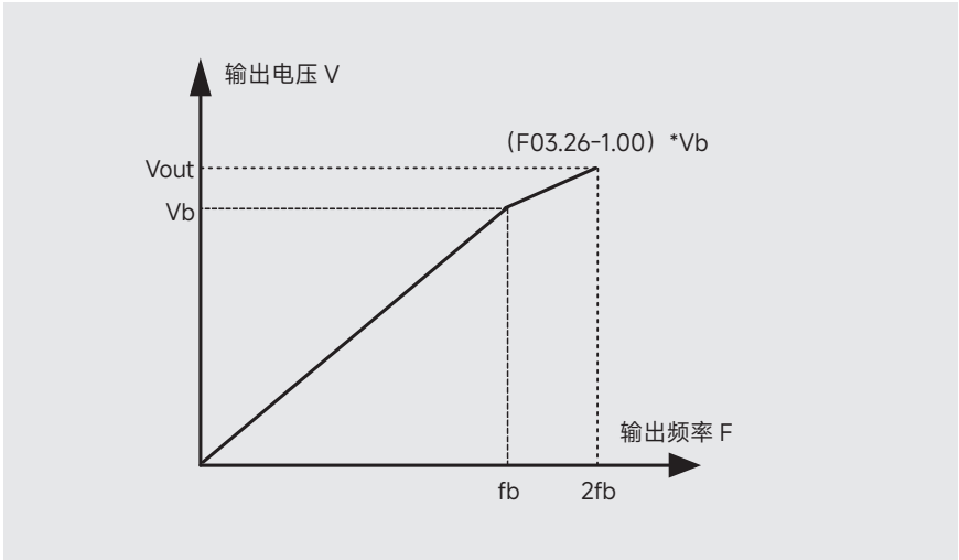
图 6-7 恒功区弱磁系数曲线图
