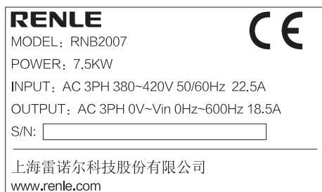
图 2-2 产品铭牌
