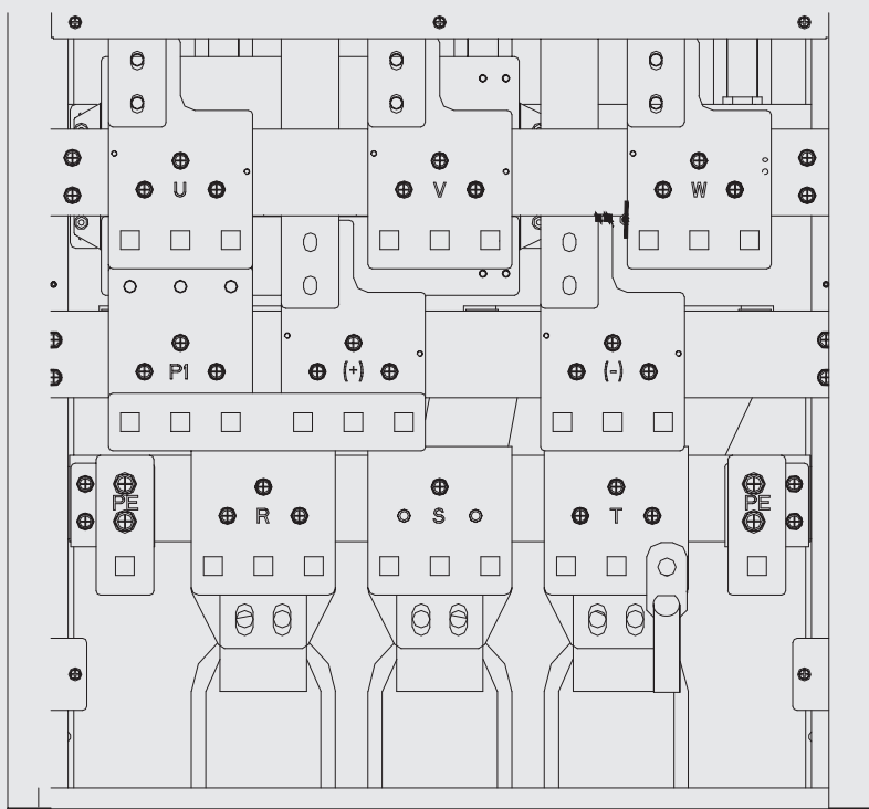
图 3-6 RNB5400-6T ~ RNB5800-6T 主回路接线端子图
