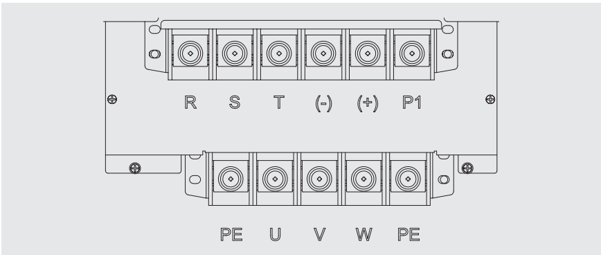
图 3-3 RNB5055-6T ~ RNB5132-6T 主回路接线端子图
