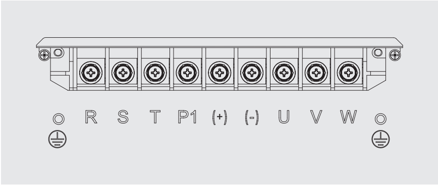
图 3-2 RNB5022-6T ~ RNB5045-6T 主回路接线端子图
