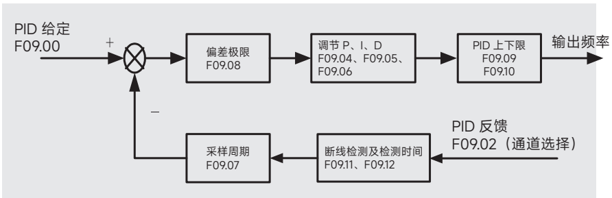
图 6-15 过程 PID 控制流程
