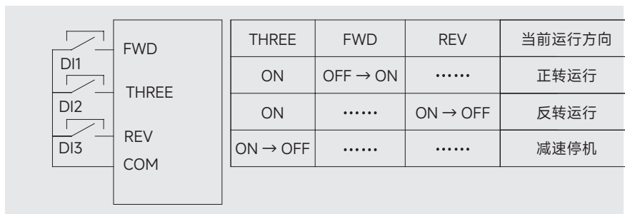
图 6-12 三线式控制 2
