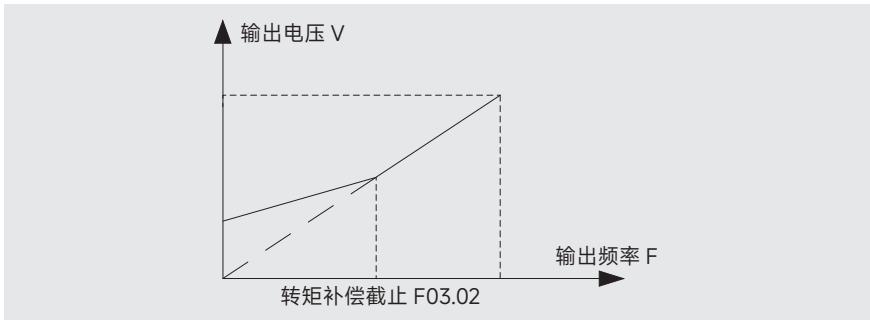
图 6-5 转矩补偿图
