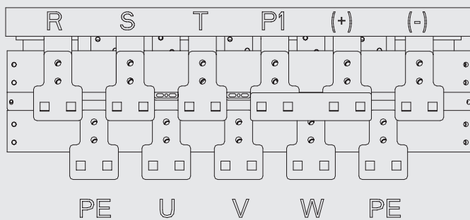
图 3-5 RNB5250-6T ~ RNB5355-6T 主回路接线端子图
