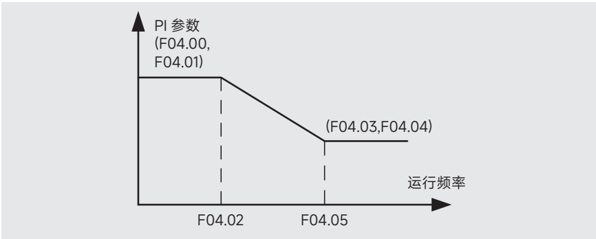
图 6-8 PI 参数与运行频率关系图
