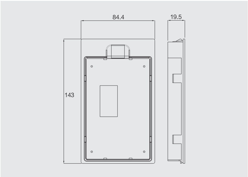
图 2-5 面板支架外形尺寸图
