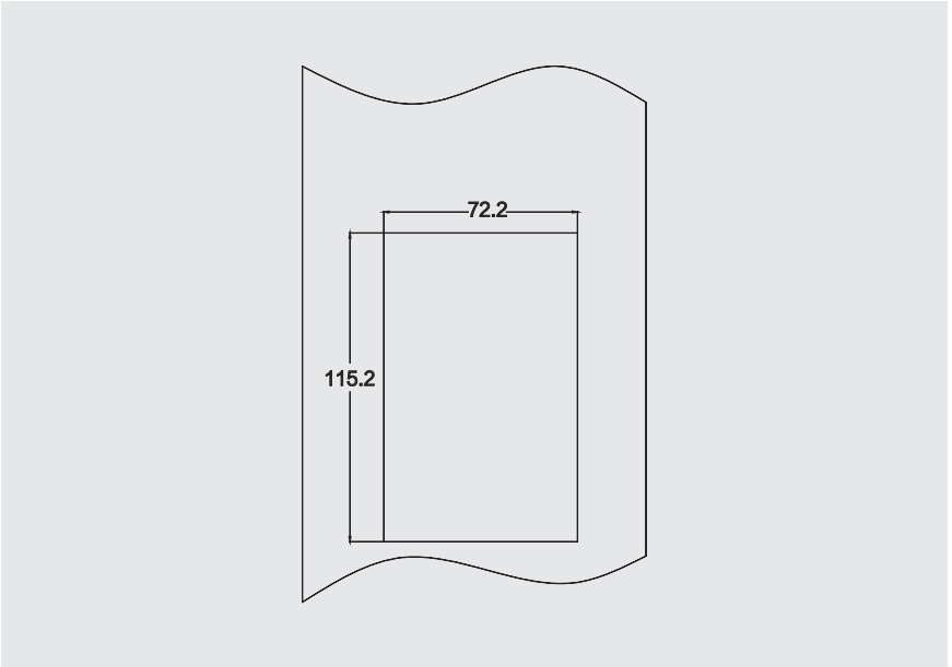
图 2-6 操作面板本体外引开孔尺寸图
