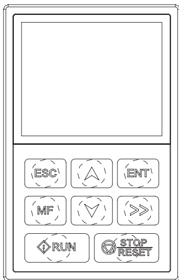
图 4-1 操作面板图
