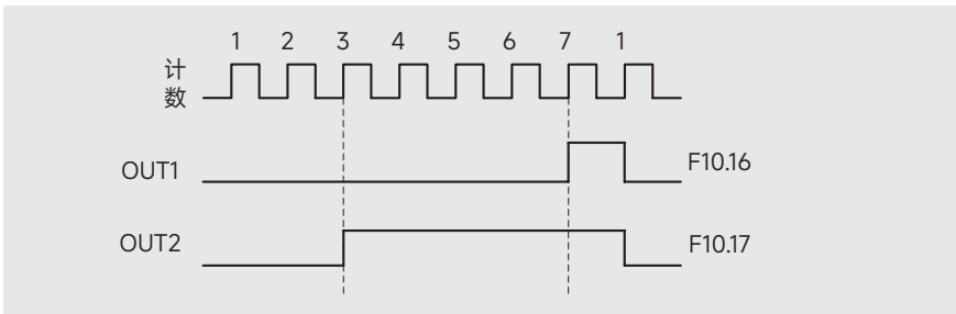
图 6-19 指定计数值与设定计数值
