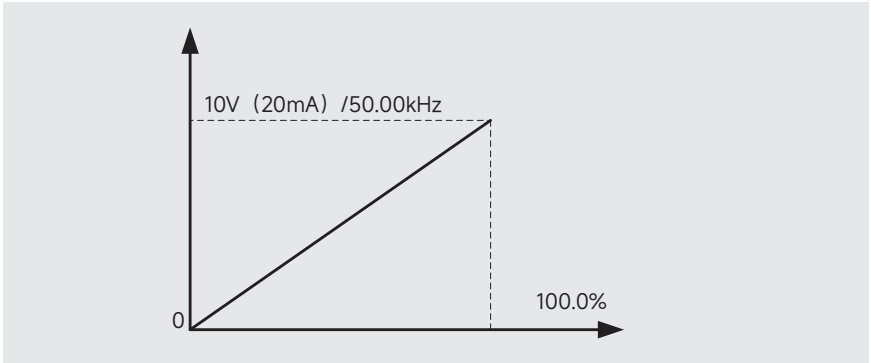
图 6-14 模拟量与高速脉冲输出对应关系
