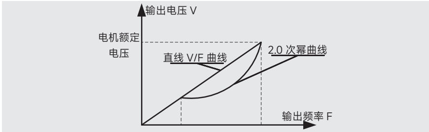
图 6-4 V/F 曲线图
