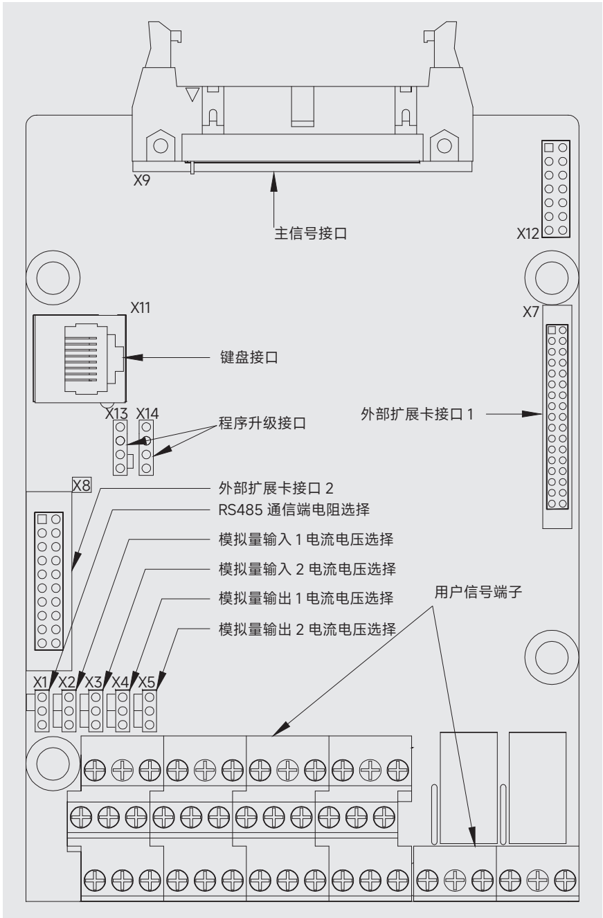
图 3-8 控制板示意图
