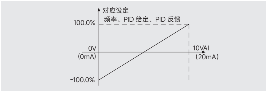
图 6-13 模拟量输入与设定值的对应关系
