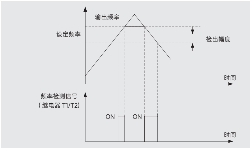
图 6-21 频率到达检测示意图
