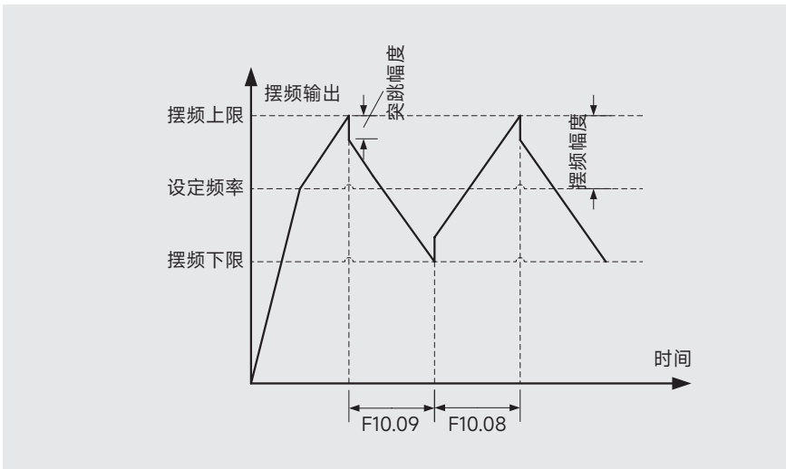
图 6-18 摆频运行
